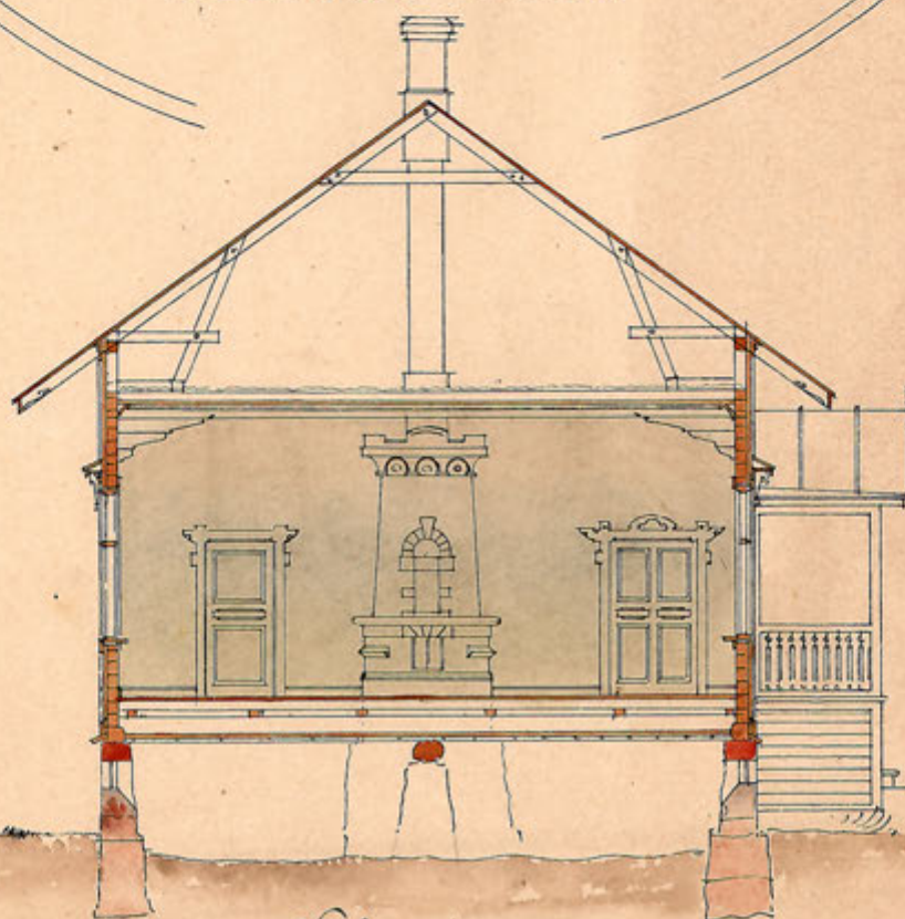
LEIKKAUS A-B
